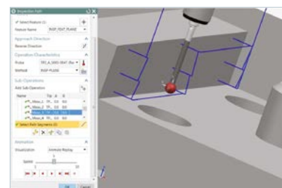
Mit NX CMM werden automatisch Prüfpfade an die Formelemente benachbarter Teile angepasst.
