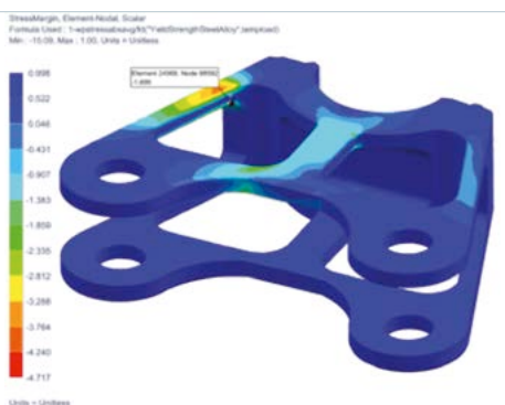
Spannungsrandberechnung basierend auf temperaturabhängiger Spannung
