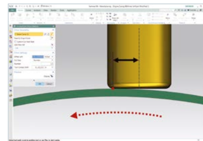
Durch die exakte Steuerung des Kontaktpunkts können die Schnittbedingungen optimiert werden.
